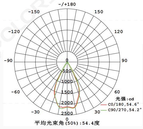
圆形格栅 55°
